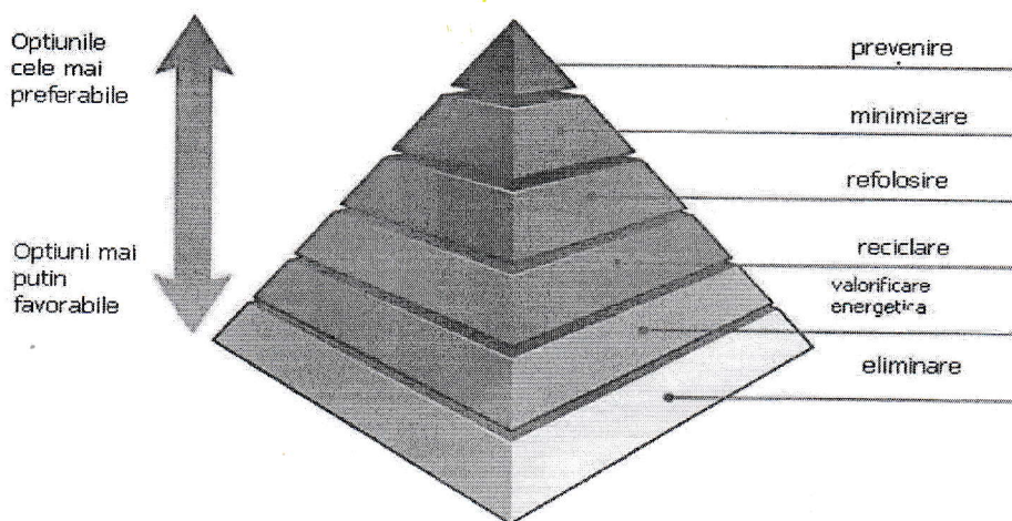
Fig.1 Ierarhia deșeurilor
